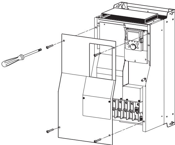
例如：ATV71HD75N4
