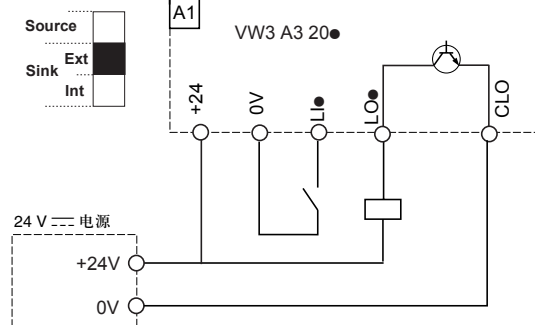
SW3 或 SW4
