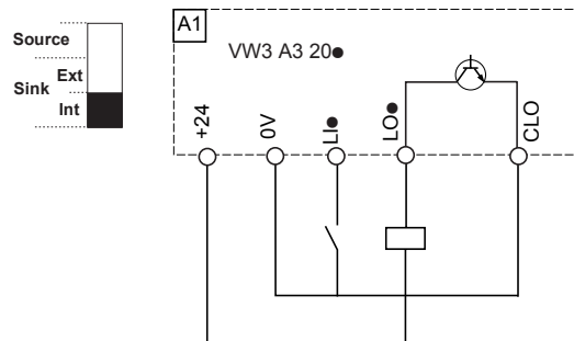
SW3 或 SW4
